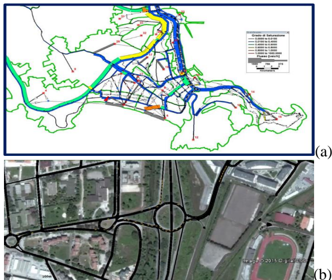
Figura n. 3. – Alcune applicazioni di modellazione della domanda di trasporto sviluppate presso l'Università degli Studi di Cassino. Distribuzione dei flussi di traffico restituita da
