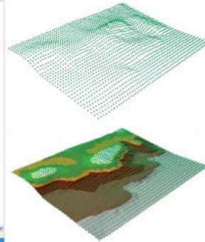
Fig. n. 4. Comune di Minturno. Creazione del DTM mediante i dati matrix, maglia 10x10m. Interpolazione e modellazione dei punti.
