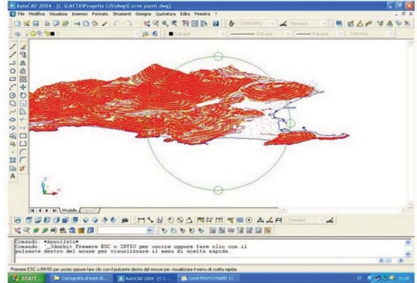
Fig. n. 4. Comune di Minturno. Creazione del DTM mediante i dati matrix, maglia 10x10m. Interpolazione e modellazione dei punti.
