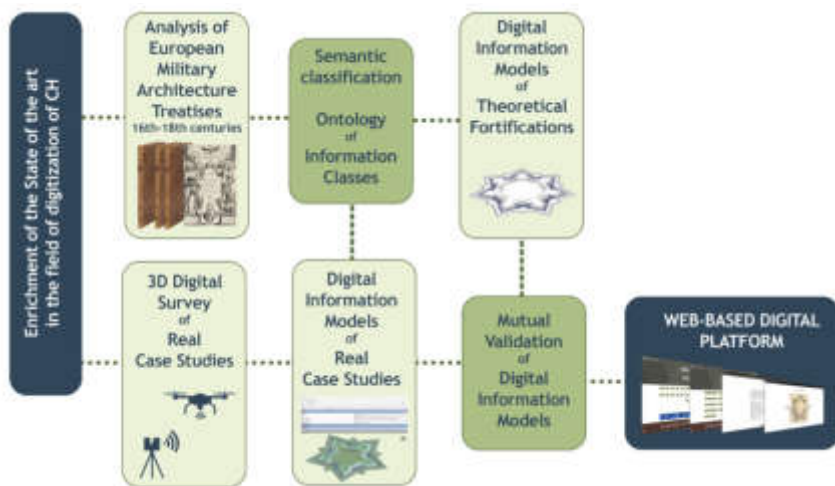
Fig. 2 - Methodological workflow (M.G. Bevilacqua, R. Spallone, A. Giordano, M. Russo).
