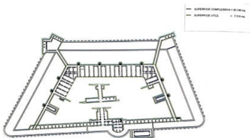
Fig. 4 - Roma, Forte Antenne, Pianta delle murature.
