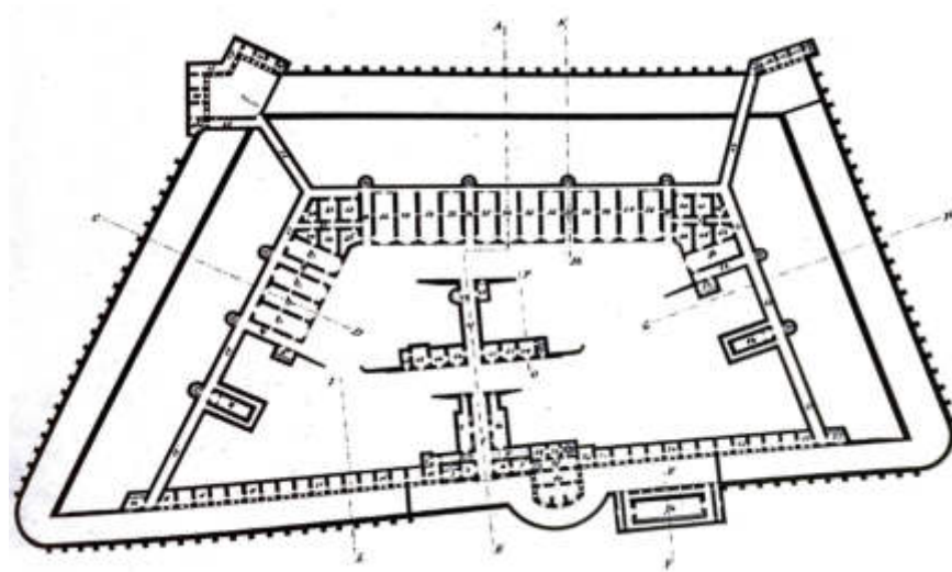
Fig. 1 - Forte Antenne, Pianta delle murature (Source: ISCAG; FT, 79B, 5264, Roma 1889, Tav. III)
